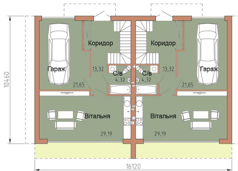
План 1-ого поверху
