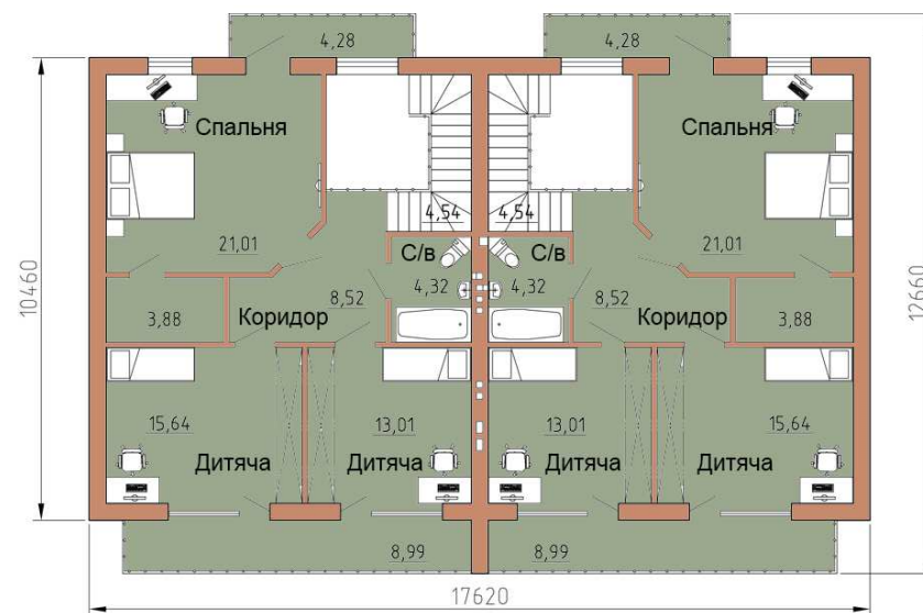
План 2-ого поверху
