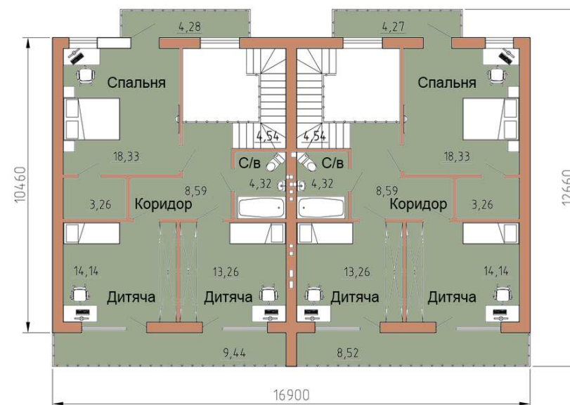
План 2-ого поверху
