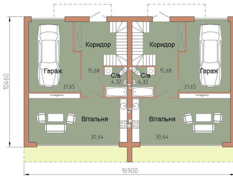
План 1-ого поверху
